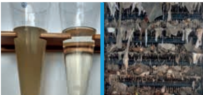
Die beiden Imhoff Trichter zeigen den Zustand der Wasserqualität. Links ist der Zulauf zum Vorklärbecken aufgefangen, der den Grobrechen passiert hat. Rechts eine Probe des gereinigten Wassers, wie es in den Vorfluter Ammer gelangt.
